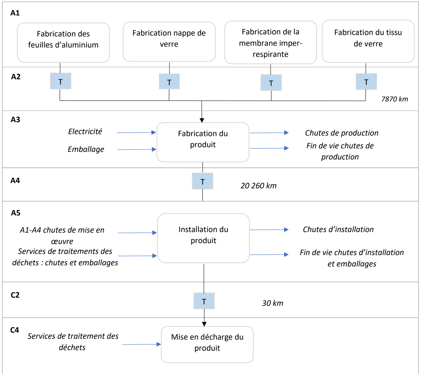
Figure : 1 : Cycle de vie de FASSATECH.
