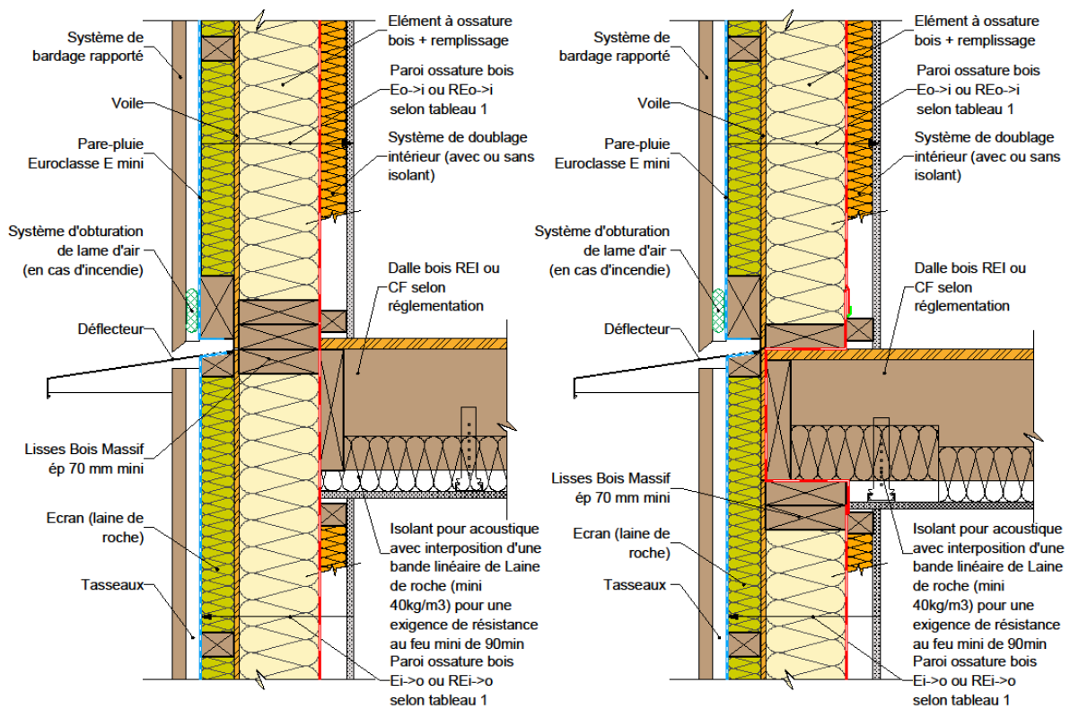
Figure 23 : Façade/mur ossature bois & plancher en ossature bois.
