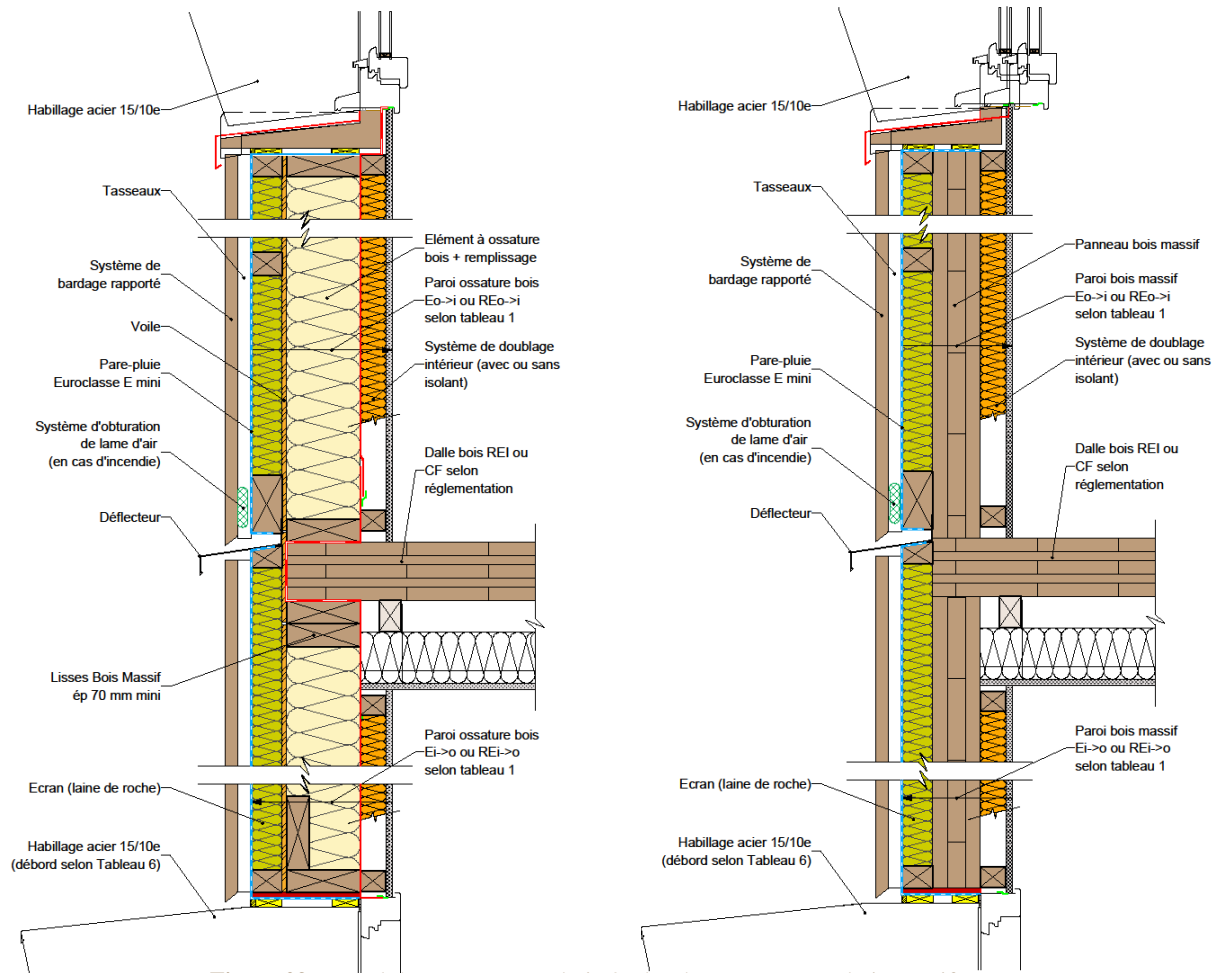
Figure 29 : Façade/mur en ossature bois & plancher en panneaux bois massif.
