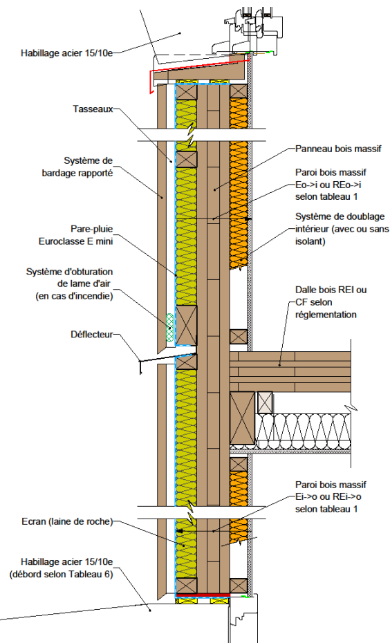
Figure 30 : Façade/mur en panneaux bois massif & plancher en panneaux bois massif.
