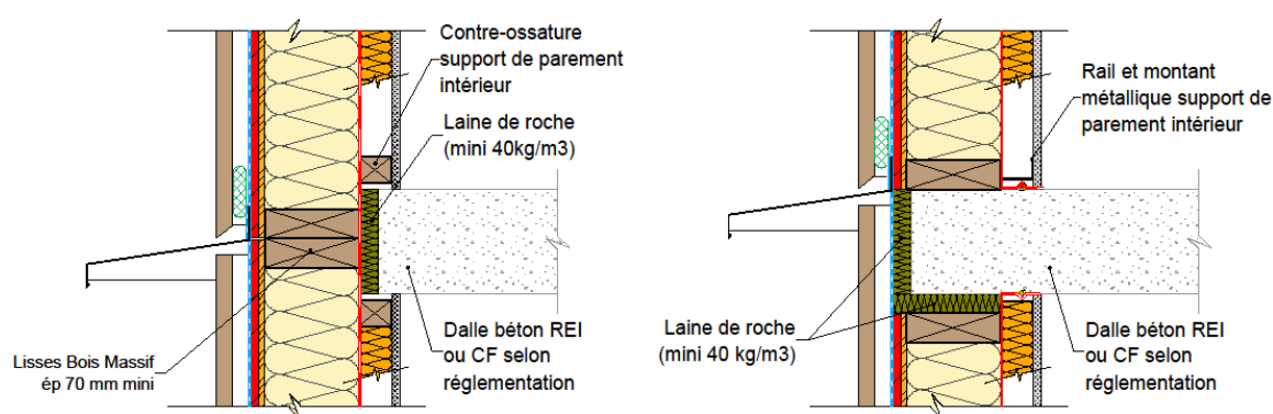
Figure 1: Traitement de l'étanchéité au nez de dalle béton (si la durée de résistance au feu de la structure est inférieure ou égale à 60 minutes).
